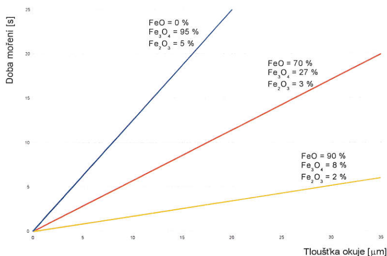
Obr. 7: Závislost doby moření na složení okuje.
