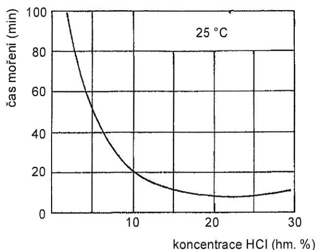
Obr. 8: Závislost doby moření na koncentraci kyseliny solné.
