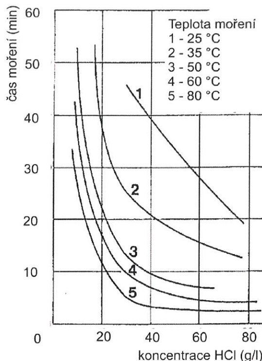
Obr. 9: Závislost doby moření na koncentraci kyseliny solné.
